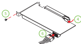
图2-10 显卡安装
