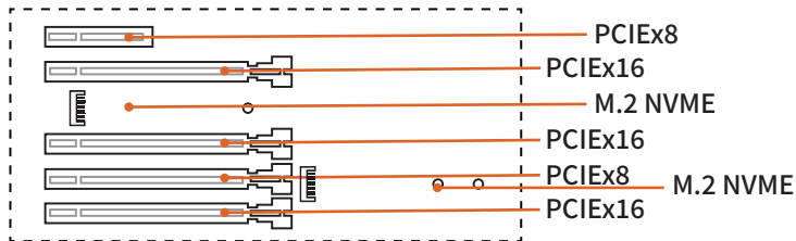
图2-3 PCI扩展插槽
