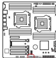
图2-3 PCI扩展插槽
